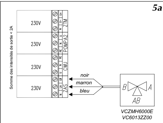
Figure 5a Schéma de raccordement de la vanne Honeywell
