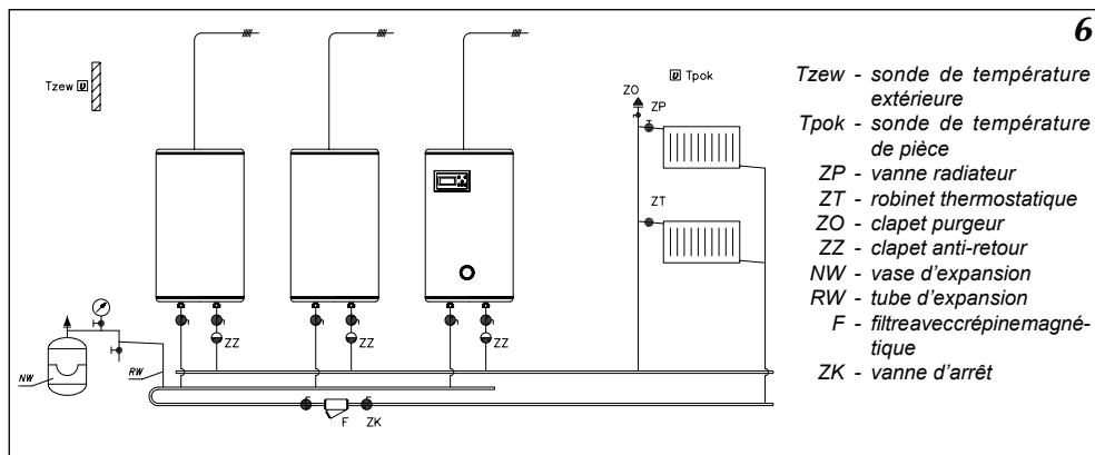
Figure 6 Raccordement de plusieurs chaudières en cascade
