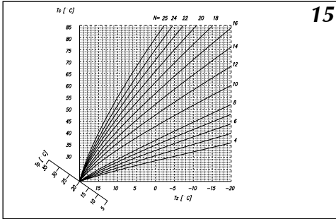
Figure 15 Courbe de chauffe
