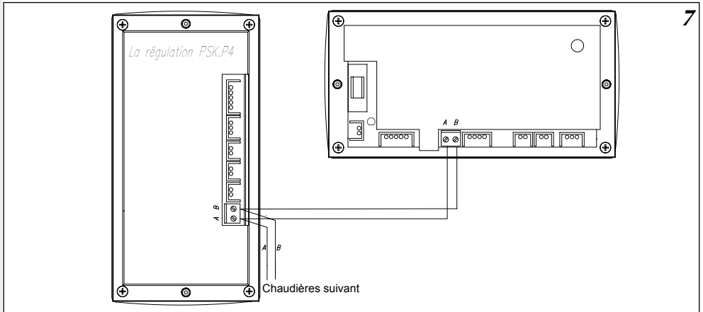
Figure 7 Branchement électrique groupe de chaudières pour fonctionnement en cascade
